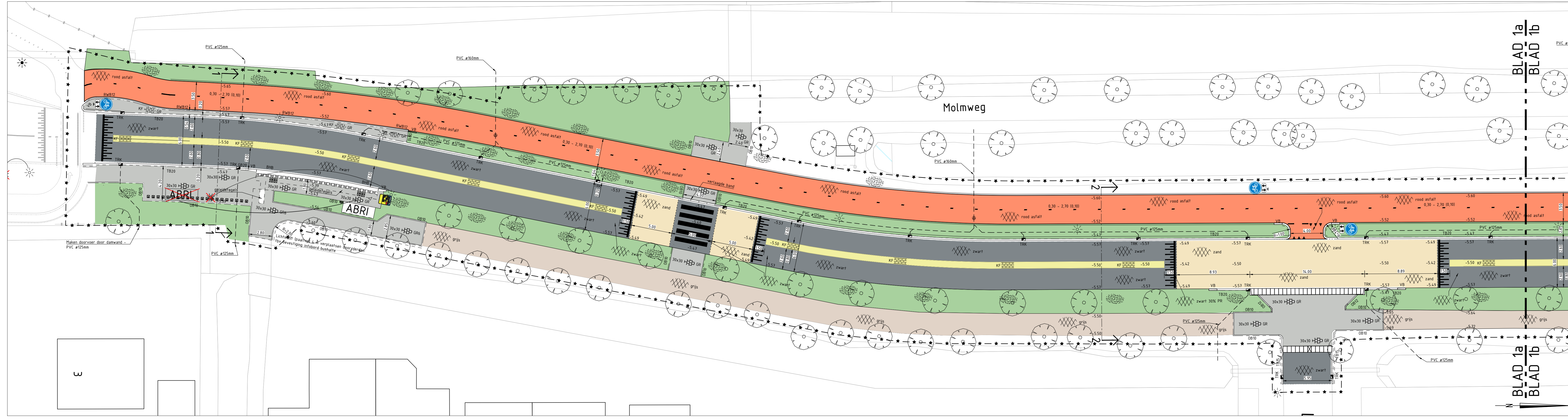
BLAD 1a SCHAAL 1:200
